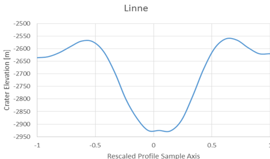
Фигура 5. Профил запад-изток (W-E) на кратера Linne, извлечен от WACGLD100. Хоризонталната ос е преместваща се за целите на следващото апроксимиране чрез полиномите на Чебишев. Формата на кратера се счита за добре запазена след формирането и като много добър пример за тип „обикновени“.
