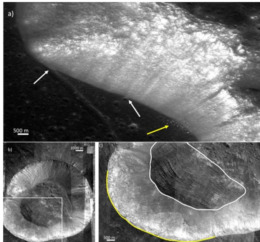
Фигура 1. а) „slump“ по дължината Promontorium Laplace, депозита е покрил малък кратер и канал (бели стрелки). Следи от боулдъри и техните след от ями (жълти стрелки) б) Срината стена на кратера Tharp; короната (в жълто) и депозита (в бяло) ясно отличими.
