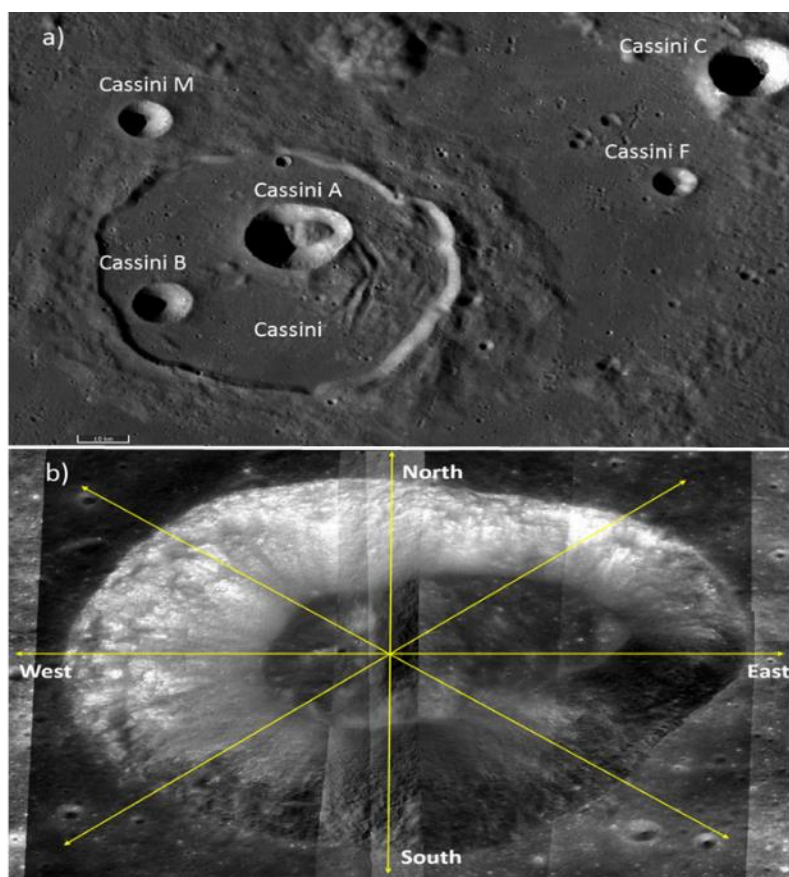
Фигура 6. а) Мозайка получена от LROC-WAC показваща кратерното семейство Cassini; б) Мозайка получена от LROC-WAC показваща кратера Cassini A; жълтите линии показват позициите на напречните сечения необходими за анализа чрез полиномите на Чебишев.
