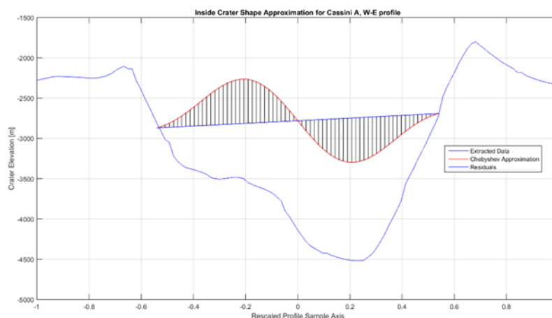
Фигура 8. Сечение Запад-Изток на Cassini A. Синията линия показва елевационния профил получен директно от WACGLD100 DEM; Червената линия показва апроксимацията на кратерната форма чрез полиномите на Чебишев използвайки M=26 уравнения, означаващи максимална степен 25; Черните линии представляват остатъците.
