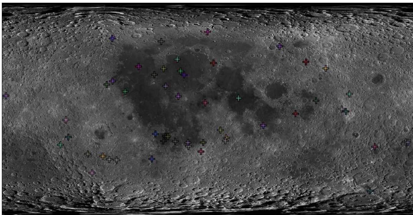
Фигура 9. Дистрибуция на анализираните 51 кратера.
