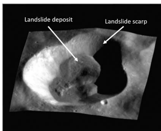
Фигура 3. Примери за свлачище от тип “slump” на Луната. Белите стрелки показват основните признаци на свлачището (т.е., откоса и депозита).
