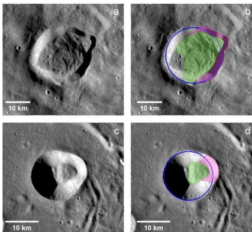
Фигура 4. Примери на свлачища в кратери. Фигури a) и b) представляват кратер Gerasimovich D; (c) и (d) Cassini A. Синята окръжност представлява кръглице била на кратер; розовите и зелените зони показват откоса на свлачището и депозирания материал:
