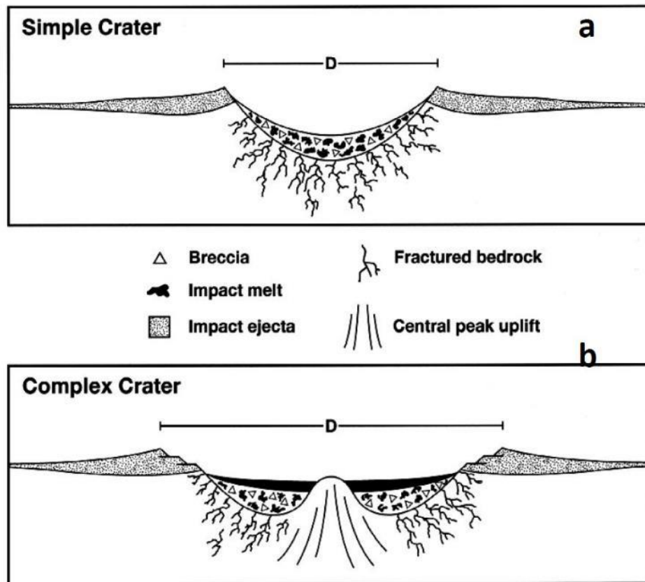
Фигура 2. Структура на а) обикновен и б) сложен кратер. (Източник: NASA)
