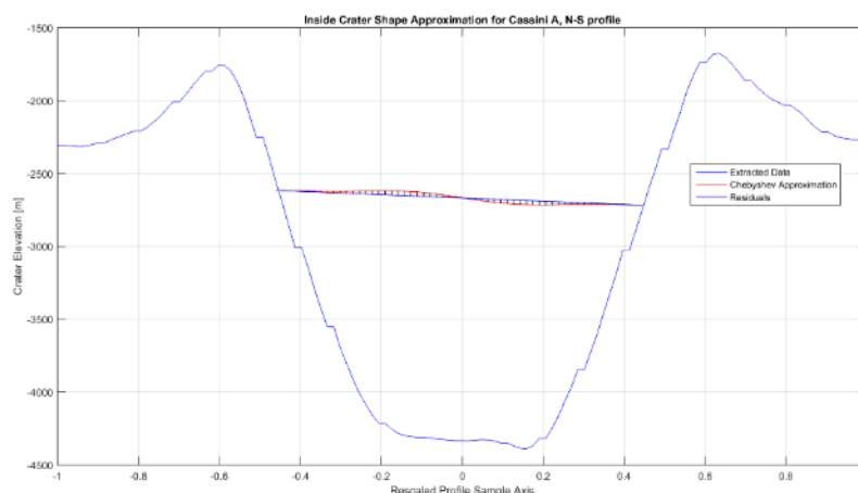
Фигура 7. Сечение Север-Юг на Cassini A. Синията линия показва елевационния профил получен директно от WACGLD100 DEM; Червената линия показва апроксимацията на кратерната форма чрез полиномите на Чебишев използвайки M=26 уравнения, означаващи максимална степен 25; Черните линии представляват остатъците.
